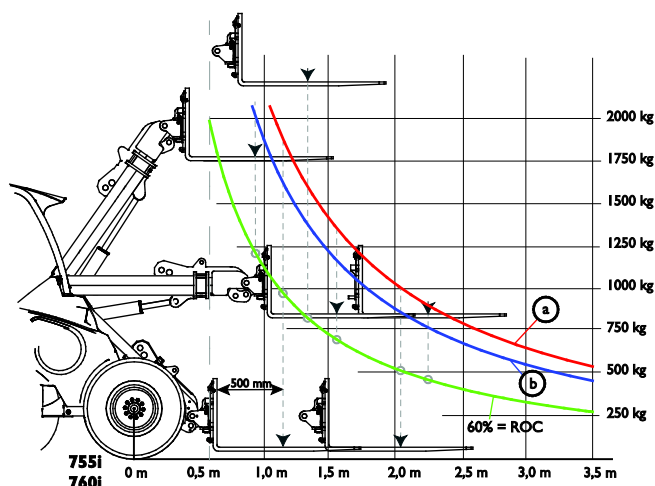
Diagram zaťaženia 755i / 760i
